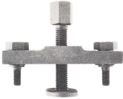
Fan puller for 1500-1600
