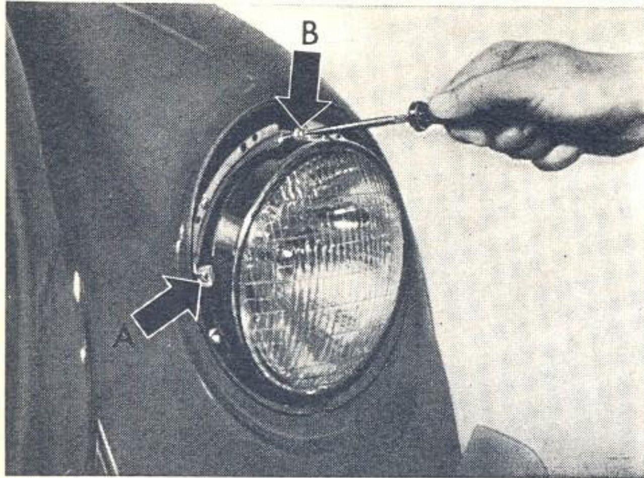
A - Ajuste lateral B - Ajuste de altura
